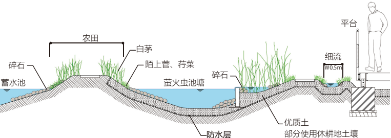
a-a' section
