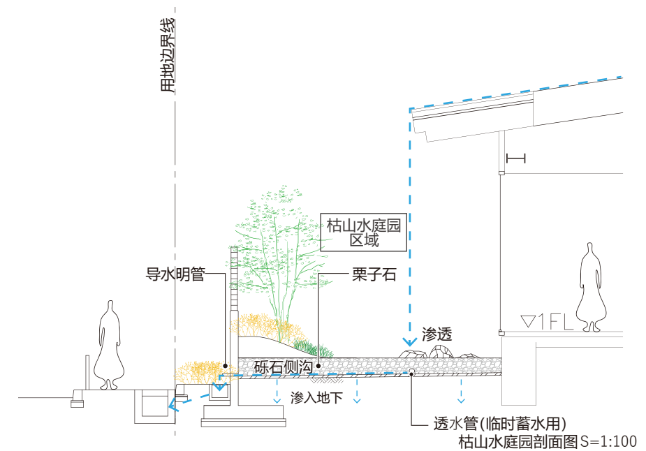
枯山水庭园剖面图 S=1:100
