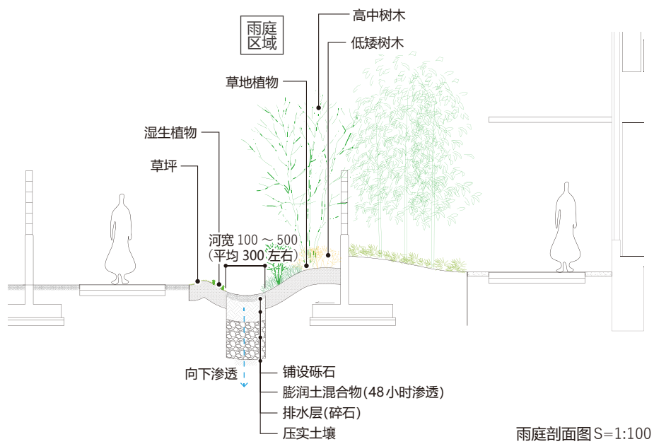
雨庭剖面图 S=1:100
