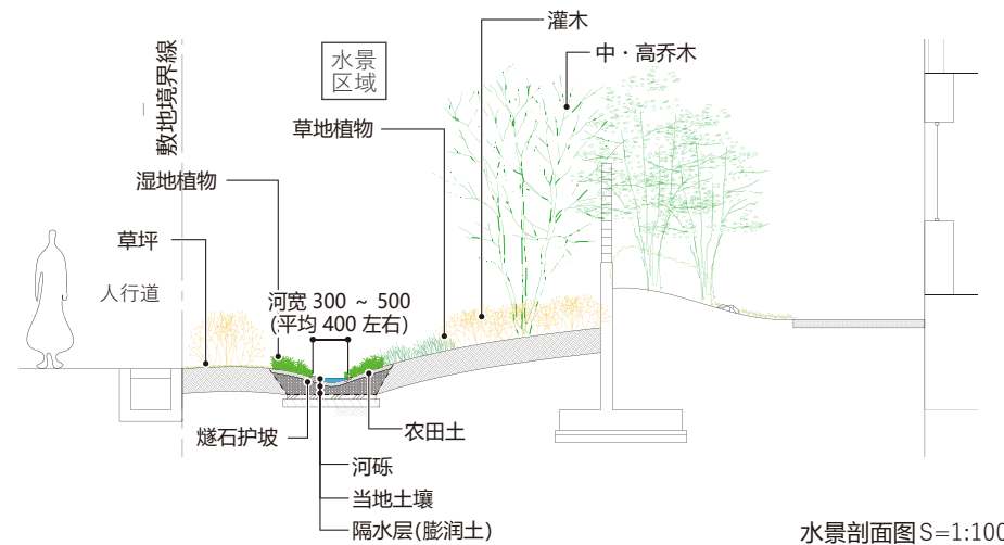
水景剖面图 S=1:100
