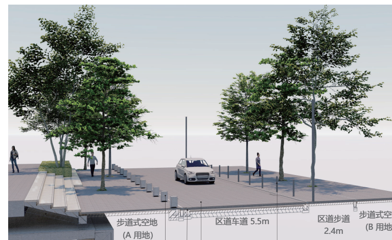
步道式空地 (A 用地) 车档兼照明 (A 用地负责) 隐藏式排水设施 区道车道 5.5m 统一铺装 区道步道 2.4m 步道式空地 (B 用地) H800 简约样式的圆柱型车档
